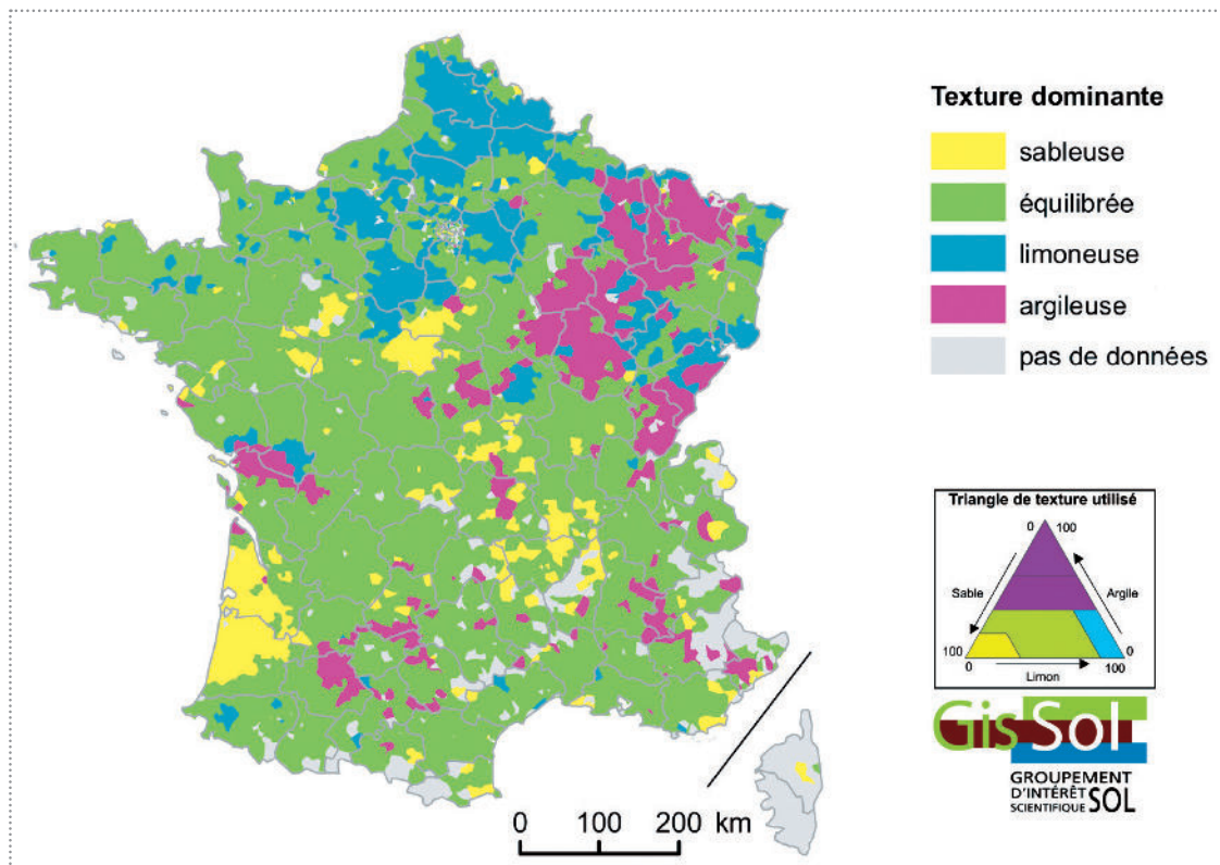
Cartographie de la texture dominante de l'horizon supérieur des sols agricoles par canton (source : BDAT).
