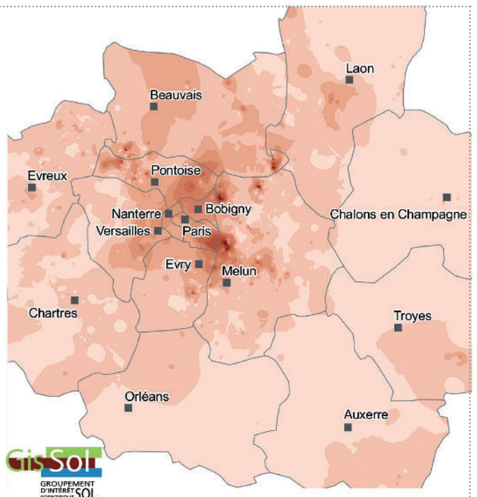
Cartographie de la distribution du mercure dans les horizons de surface du Bassin parisien (source : BDETM).
